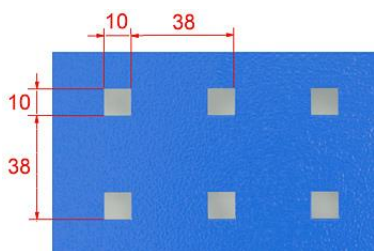
Wymiary perforacji
